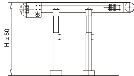
Abstützung Typ 2
