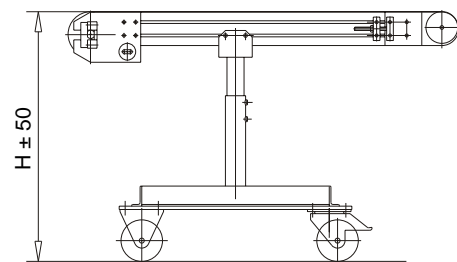
Abstützung Typ 4
